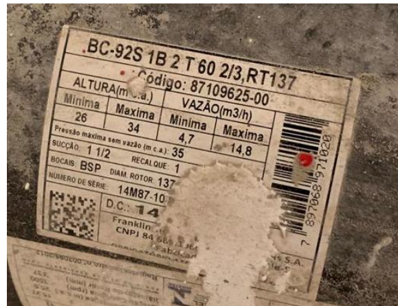
Especificações moto-bomba
